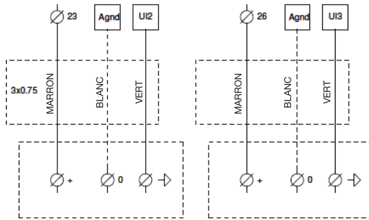
Soufflage LOBBY
