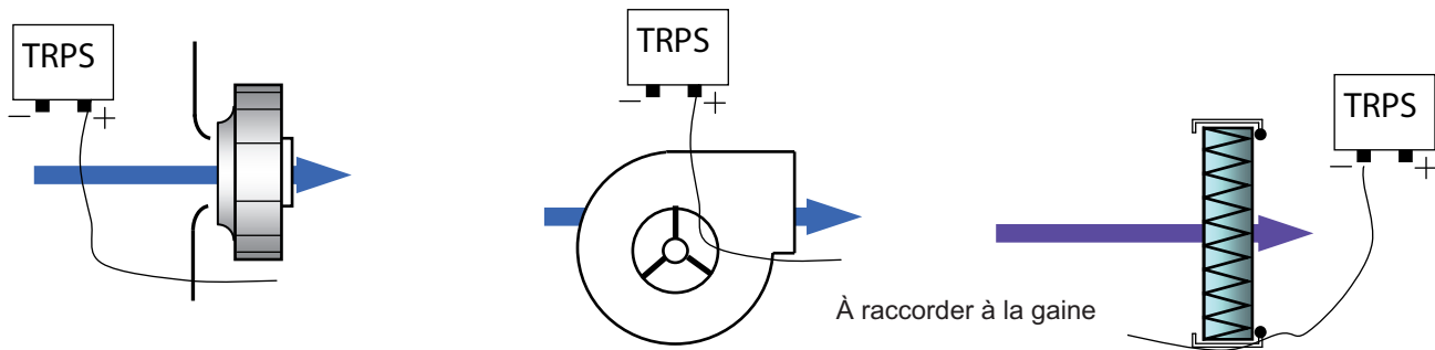
Soufflage LOBBY
